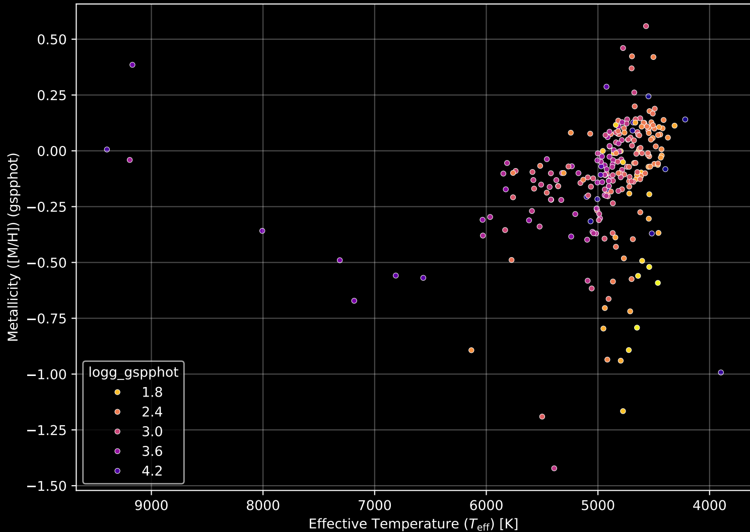
APOGEE DR17 Field: [005+12] Stellar Population Parameters (n= 247)
